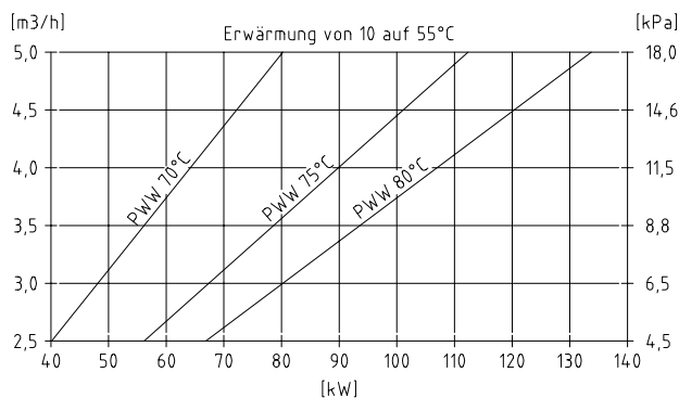
Leistungs- und Druckverlustdiagramm
