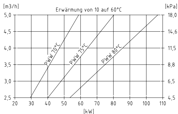
Leistungs- und Druckverlustdiagramm
